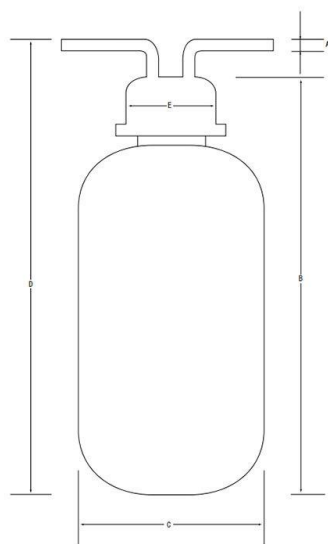
■外形尺寸法图
